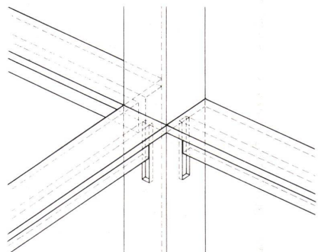
3 Stütze der Eisenkonstruktion. Gezogenes Vierkantrohr 40/40 verzinkt mit zweiseitig eingesetzten Wandplatten. Verbindung durch Haken, die in Stützenschlitz greifen. Die Stützen sind durchgehend auf vier Seiten im Abstand von 50 cm geschlitzt.
