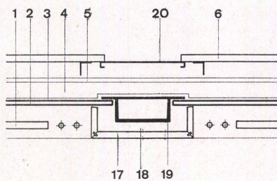
Horizontalschnitt durch Brüstung und Nebenstütze 1:15. Section horizontale à travers allège et pilier secondaire. Horizontal section of parapet and second- ary support.
