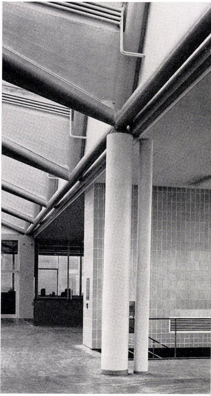
1 Stützensbildung der 60 m weit gespannten Stahlkonstruktion im Flachbau. Stahlrohr-Pendelstütze mit dahinter liegendem Regenfallrohr.
