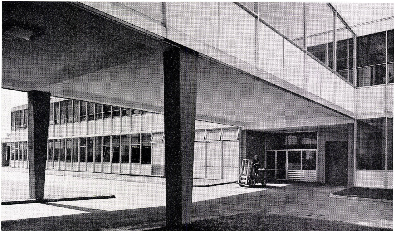
3 Verbindungsbrücke vom Geschößbau zum Flachbau. Vorgehängte Fassade mit weißen, emailierten Brüstungen.
