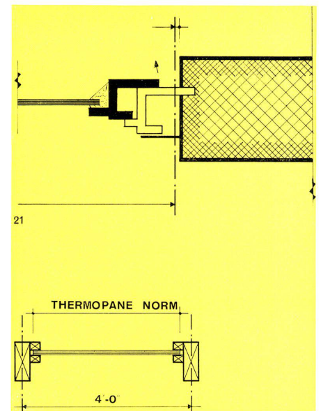
21 und 22 Normierte Stahlfensterrahmen. Der Wunsch nach Unabhängigkeit von der anschließenden Konstruktion führt zu einer Verbreiterung des Rahmens.
