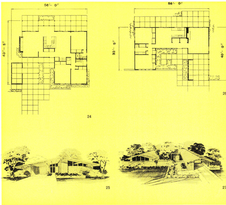
24-27 Teilweise vorgefertigte Häuser, nach Modulordnung vermaßt und konstruiert. Maisons en partie préfabriquées, cotées et construi- tes d'après une trame. Partly prefabricated houses dimensioned and con- structed on a modular principle.
