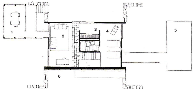
1 Grundriß des Sonnenhauses 1:250 1 Sitzplatz 2 Wohnraum 3 Ankleideraum 4 Elternschlafzimmer 5 Automobilstand 6 Sonnenkollektor
