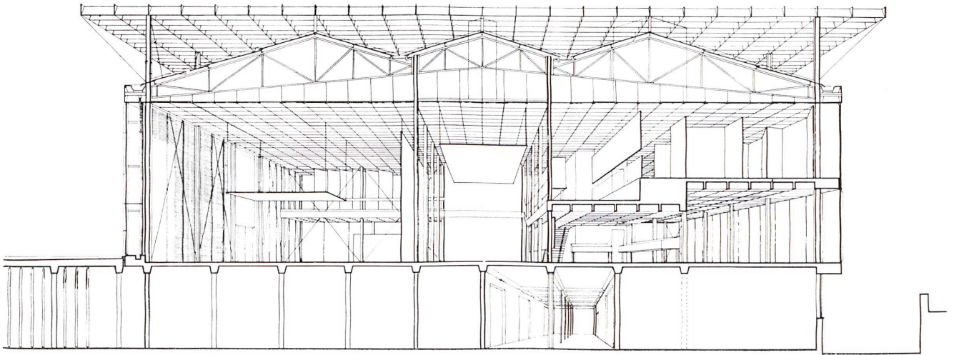
4 Querschnitt durch das ganze Gebäude. Coupe transversale sur l'ensemble du bâtiment. Cross section of the entire building.
