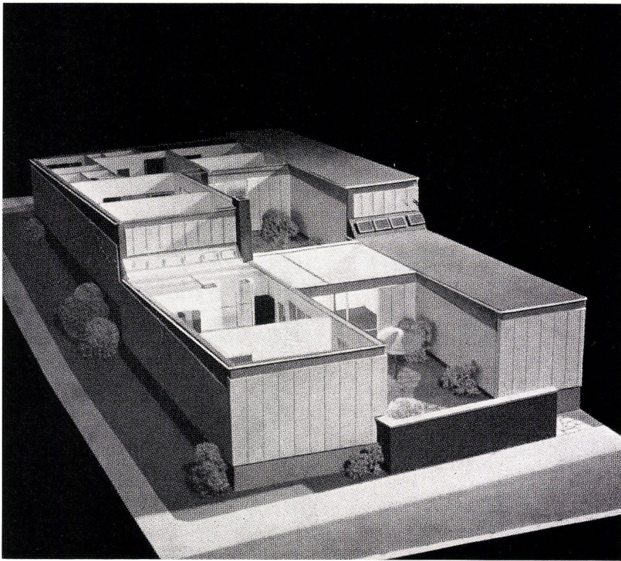
Gestaffelte Teppichhäuser mit 3 und 4 Zimmern. (Im Lageplan «W») Maisons individuelles à échelonnage caractéristique avec 3 et 4 pièces (Dans le plan de situation «W») Grading-type single family houses with 3 and 4 rooms (In the site plan "W")
