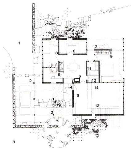
1 Einfahrt / Entrée pur voitures / Drive-way 2 Gedeckter Autounterstand / Abri couvert pour voitures / Covered car shelter 3 Hof mit Pergola / Cour avec pergola / Yard with pergola 4 Hauseingang / Entrée de la maison / Main entrance 5 Eingang, Garderobe / Entrée, vestiaire / Entrance, cloakroom 6 Spielzimmer / Salle de jeux / Game room 7 Schreibplatz / Coin-bureau / Study corner 8 Zimmer mit Kajütenbetten / Pièces avec lits-cabine / Room with bunks
