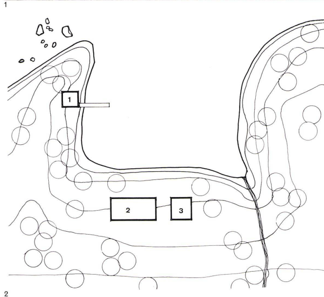
2 Lageplan 1:1000. Plan de situation. Site plan. 1 Sauna 2 Ferienhaus / Maison de vacances / Vacation house 3 Doppelgarage / Garage double / Double garage
