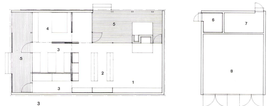
3 Ferienhaus mit Garage 1:200. Maison de vacances avec garage. Vacation house with garage. 1 Wohnraum / Séjour / Living room 2 Küche / Cuisine / Kitchen 3 Schlafzimmer / Chambre à coucher / Bedroom 4 Elternschlafzimmer / Chambre des parents / Parents' bedroom 5 Veranda 6 Keller / Cave / Cellar 7 Lager / Provisions / Supplies 8 Doppelgarage / Garage double / Double garage
