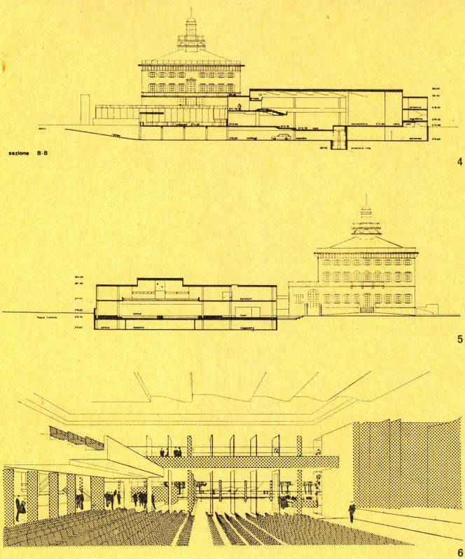
3. Preis Fr. 7750.-: Projekt 43, Kennwort Spazio, M. Rasser und T. Vadi, Basel.
