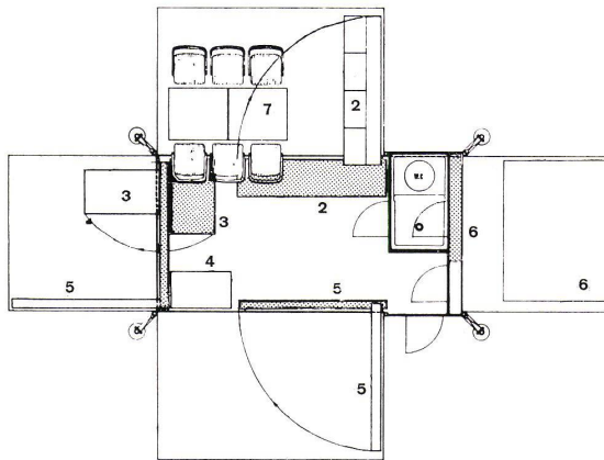
1 Der auseinandergeklappte Wohnwagen auf der Triennale. Vorn sieht man den auf den Grundrissen linken Teil mit dem Küchenelement und der an der Wand befestigten Zweibettkoje. Die Kopfseiten der vier Raumteile sind mit aufrollbarem Nylonstoff abschließbar.
