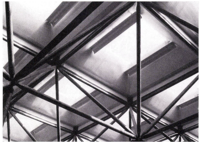
12 Die dreiseitige Anordnung der Bänke an den Altar. 13 Die Rückseite mit dem Beichtstuhl und den Schränken frei in den Raum gestellt. 14 Bauaufnahme. 15 Die Kunststoffoberlichter mit den Be- leuchtungsrohren. 16 Das räumliche Fachwerk. 17 Das Knotenstück. 18 Deckenknoten von unten.
