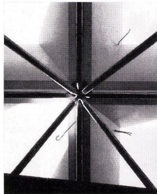
12 Die dreiseitige Anordnung der Bänke an den Altar. 13 Die Rückseite mit dem Beichtstuhl und den Schränken frei in den Raum gestellt. 14 Bauaufnahme. 15 Die Kunststoffoberlichter mit den Be- leuchtungsrohren. 16 Das räumliche Fachwerk. 17 Das Knotenstück. 18 Deckenknoten von unten.
