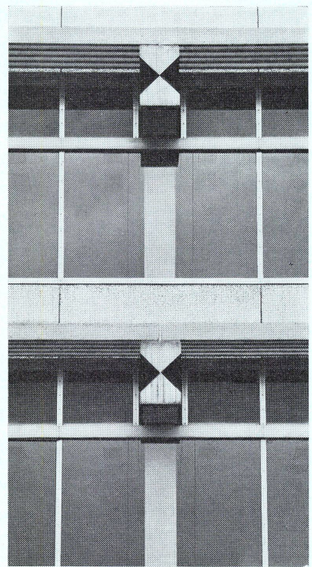
5 Ein Balkenkopf mit seiner typischen Sanduhrform, darüber die Sonnenblenden.
