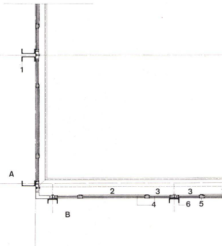
4 Schnittdetail 1:50. Détail de coupe. Section detail.
