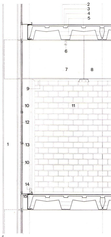
2 Fassadendetail aus einer Längsfassade mit den Doppelstahlpfeilern. Sie sind aus je zwei U NP 40 zusammengesetzt und akzentuieren die Längsfassaden mit ihrem Rhythmus. Zwischen diesen Doppelpfeilern liegt jeweils ein Belüftungselement, das in der Fassade als schwarzes Gitter erscheint. Im übrigen zeigt die Detailsansicht die selben Fenster wie an den Schmalfassaden, bestehend aus je zwei festen Scheiben und einem Fensterflügel. Über und unter diesen Fenstern sind Thermoluxverglaste Flächen.
