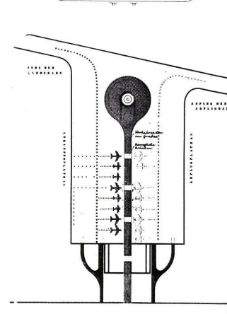
1 Paris-Orly, Paris-West. Entwurf: Aéroport de Paris. Aus «Interavia», Genf.
