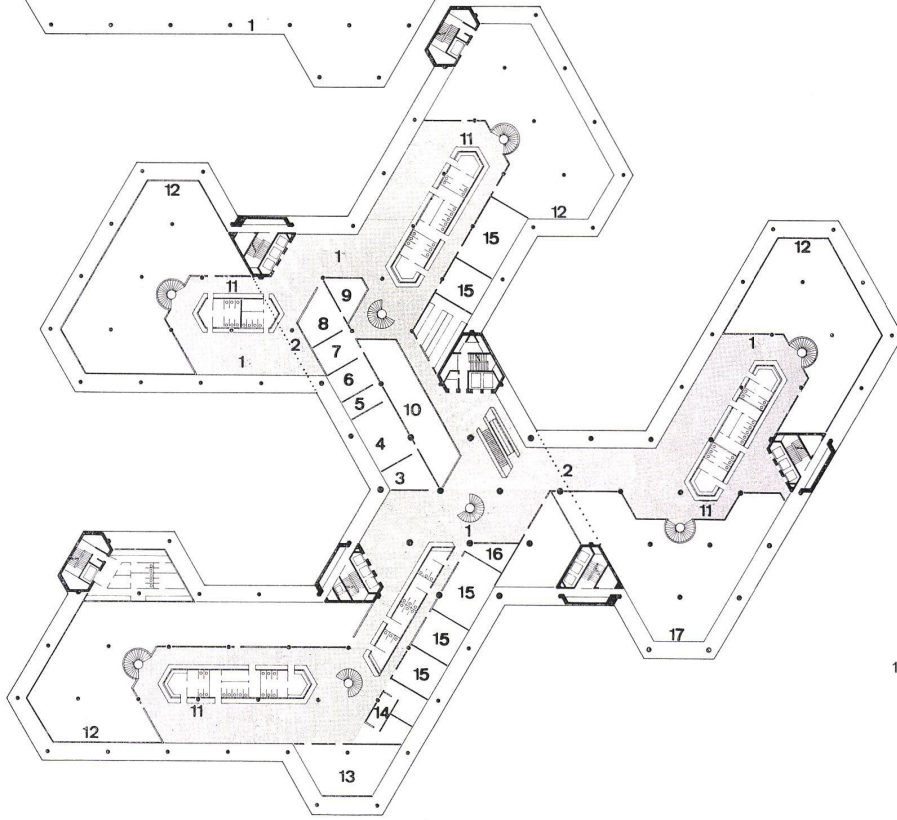
17 Hauptverwaltung der Deutschen Krankenversicherungs AG, Köln. Grundriß 2. Obergeschoß ca. 1:1000. Kraemer, Pfennig, Sieverts.
