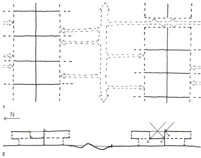
1 Schematischer Grundriß der «back-to-back»-Bebauung.
