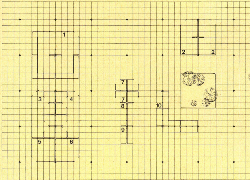
15 Großpavillon, Grundriß 1:200.
