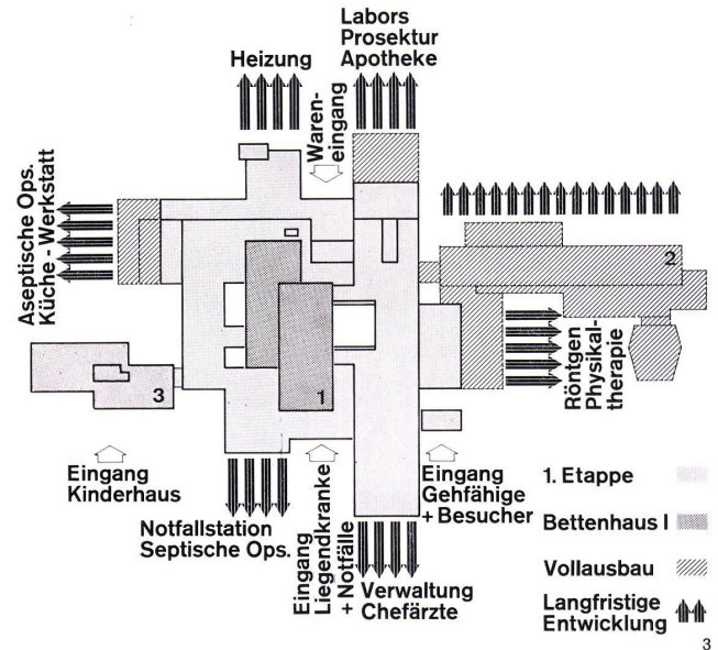
4 Behandlungsebene (Erdgeschoß) 1:1000.
