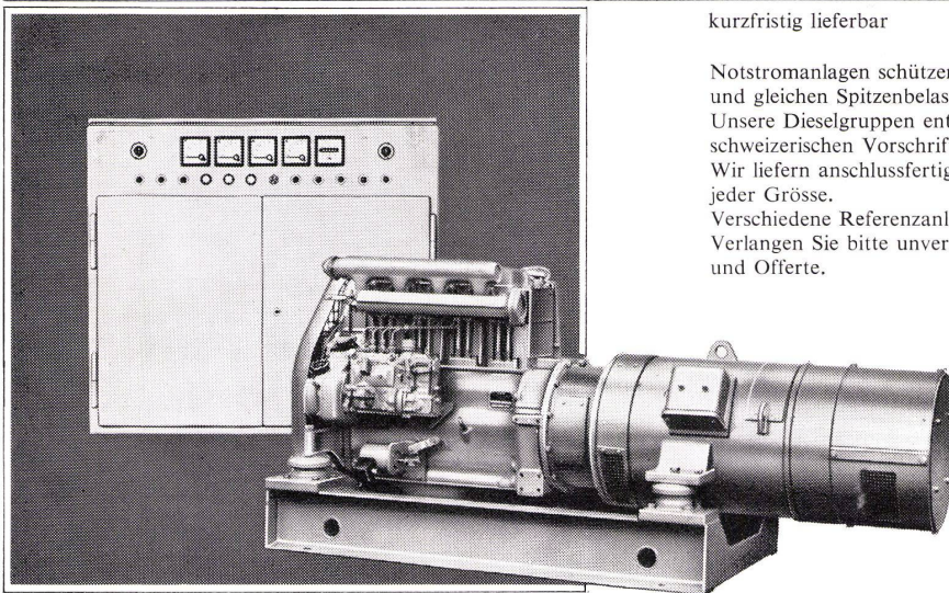
Diesel-Notstromaggregat 25 kVA, 50 Hz, 380 V mit Schaltschrank für Automatik
