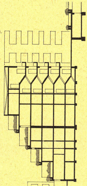
5 2. Obergeschoß 1:500.
