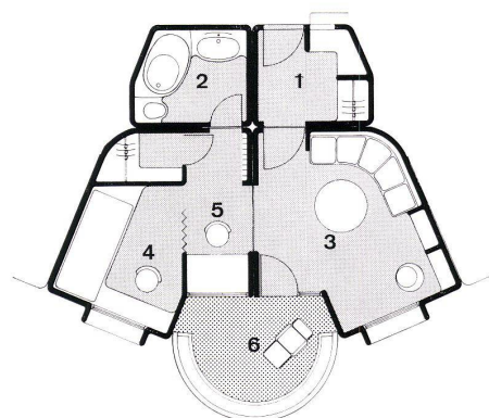
12 Grundriß 1:135. Wohnungseinheit. Plan 1:135. Unité habitable.
