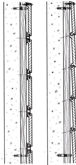
senkrechtes und waagrechtes Montagebeispiel
