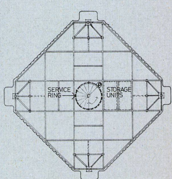
7 Strukturplan.
