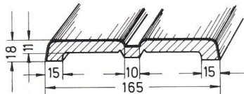
Die verschiedenen Kantenausbildungen der Bauprofile
