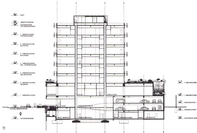
10 Querschnitt. Variable Lage der Korridorzone. Coupe transversale: La zone de circulation peut être déplacée. Cross section. Variable location of corridor zone.
