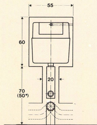
Aussparungsmasse
