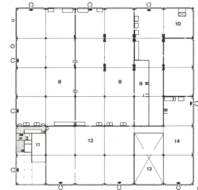
7 Grundriß Erdgeschoß. Plan du rez-de-chaussée. Plan of ground floor.
