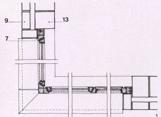
1 Schnitt A-A durch Holzgesims. Coupe A-A sur la corniche supérieure. Section A-A of wooden cornice.
