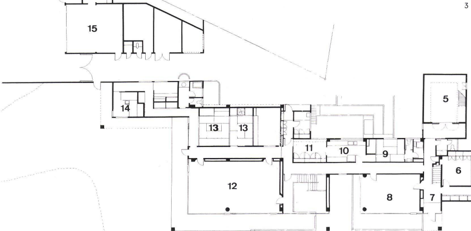
4 Erdgeschoß 1:400. Rez-de-chaussée. Ground floor. 1 Schlafrum / Chambre à coucher / Bedroom 2 Studio 3 Ankleide / Vestiaire / Dressing room 4 Luftraum des Lagerraums / Vide de la réserve de provisions / Air space above storeroom 5 Lagerraum / Réserve de provisions / Storeroom 6 Gastzimmer / Chambre d'hôte / Guest room 7 Dienstingang / Entrée de service / Service entrance 8 Wohnraum / Salle de séjour / Living room 9 Dienstenzimmer / Chambre de service / Utility room 10 Küche / Cuisine / Kitchen 11 Schrankraum / Rangement / Cupboards 12 Empfangsraum / Pièce de réception / Reception room
