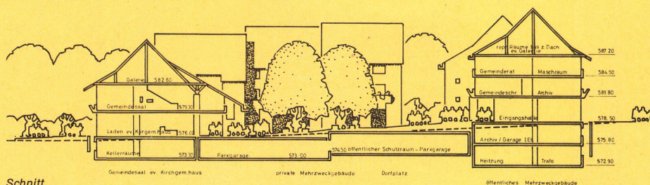
Schnitt.
