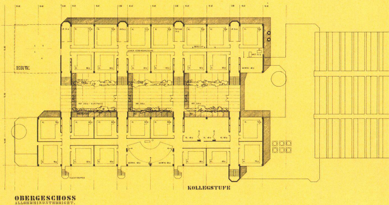
OBERGESCHOSS ALLGEMEINENTWURF
