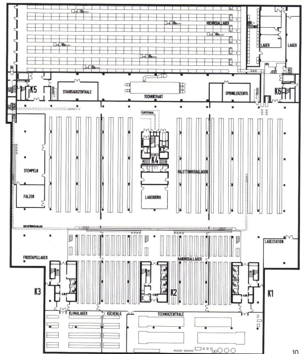
9 Grundriß Erdgeschoß 1:1200. Plan du rez-de-chaussée. Plan of ground floor.
