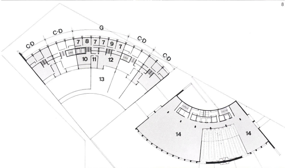
8 Grundriß 2. Obergeschoß mit Botschafterwohnung 1:1000. Plan du 2ème étage avec appartement de l'ambassadeur. Plan of 2nd floor with ambassador's quarters.
