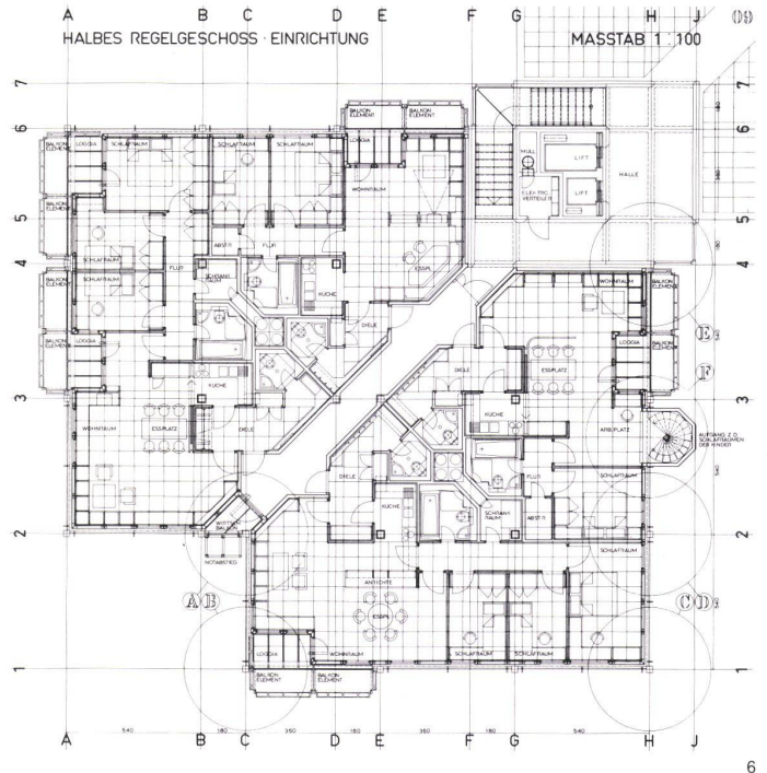
5 Axonomie. Axonomie. Axonomy. 6 Grundriß. Plan.
