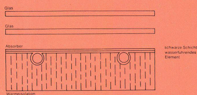
Wärmefluss im Sonnenkollektor
