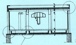
COUPE BB
