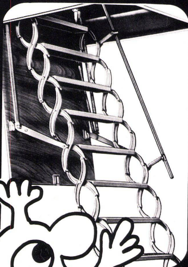
Scherentreppen
