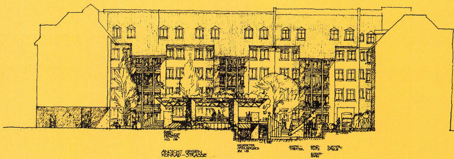
ANSICHT SÜDEN ANSICHT STRASSE
