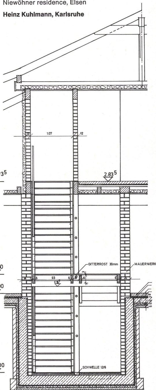
SCHNITT C-D
