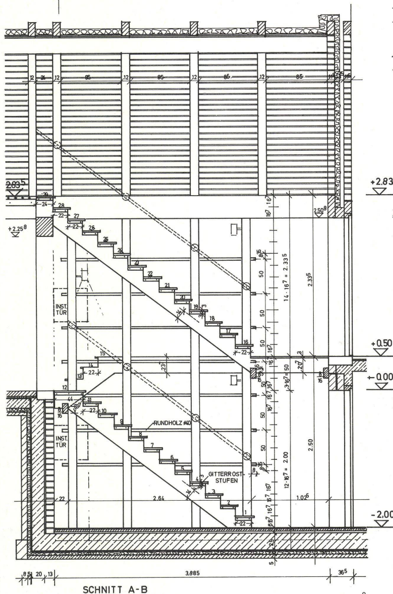
SCHNITT A-B
