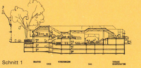
Schnitt 1
