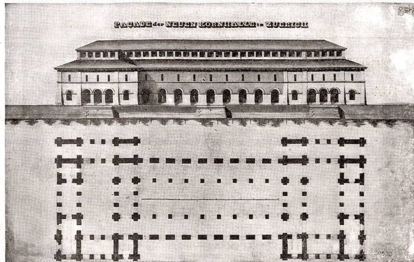
Grundriß/Auflriß zum «neuen Kornhaus» auf dem alten Tönhalleplatz, von Baumeister Johann Faller, ausgeführt 1837/39 durch Ing. Negrelli, den Erbauer der Münsterbrücke von 1836/38. Von dem aus Sufers im Rheinwald gebürtigen Faller stammt übrigens die schöne hölzerne Russener Brücke bei Disentis, wie auch das Kurhaus Schuls-Tarasap.
