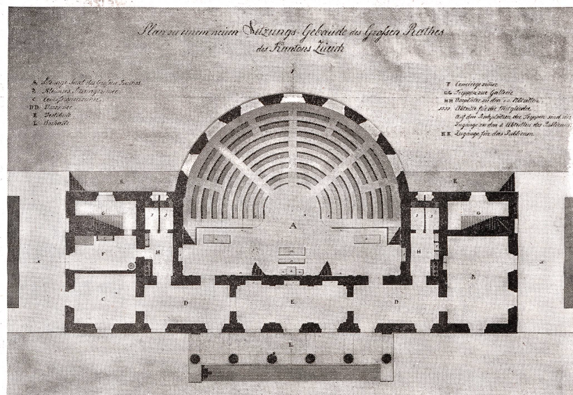
Entwurf zu einem Großratsgebäude in Zürich, 1832, Grundriß von Kaspar Vögeli, der aus einem Planwettbewerb, für den damals Fr. 400,—, 300,— und 200,— ausgesetzt wurden, den 1. Preis davontrug. Der Bau kam allerdings nie zur Ausführung, da man die hohen Kosten scheute.
