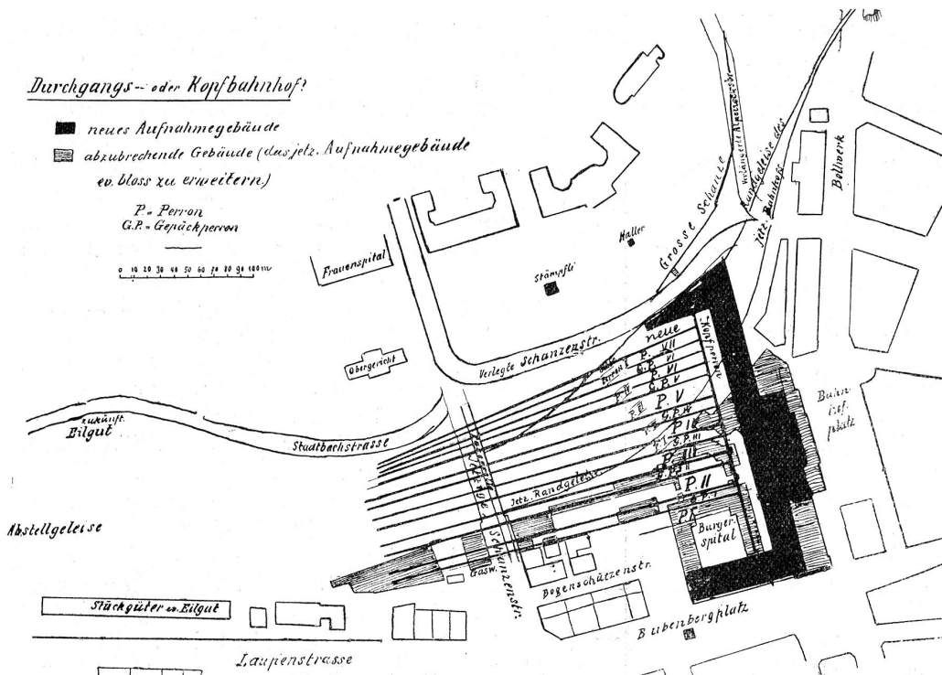
Die Berner Bahnhoffrage. Kopfbahnhof mit Geleisorientierung nach Westen.
