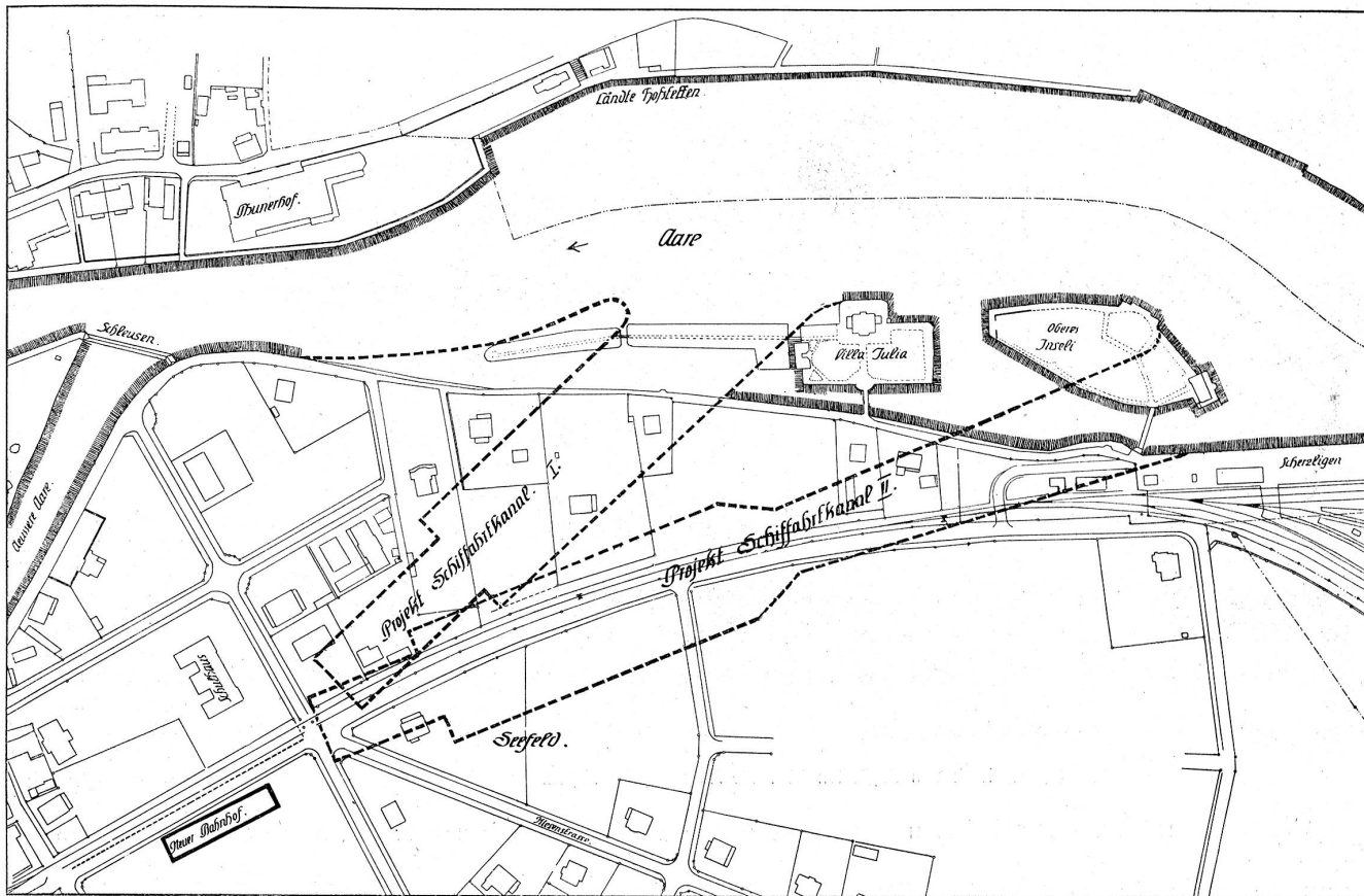
Projekte für die Erstellung eines Schiffahrtskanals als Anschluss an den Zentralbahnhof in Thun.
