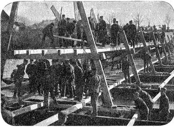
Schweizerische Militärbilder: Konstruktion einer Etagen-Schiffbrücke über den Hagneckkanal.
