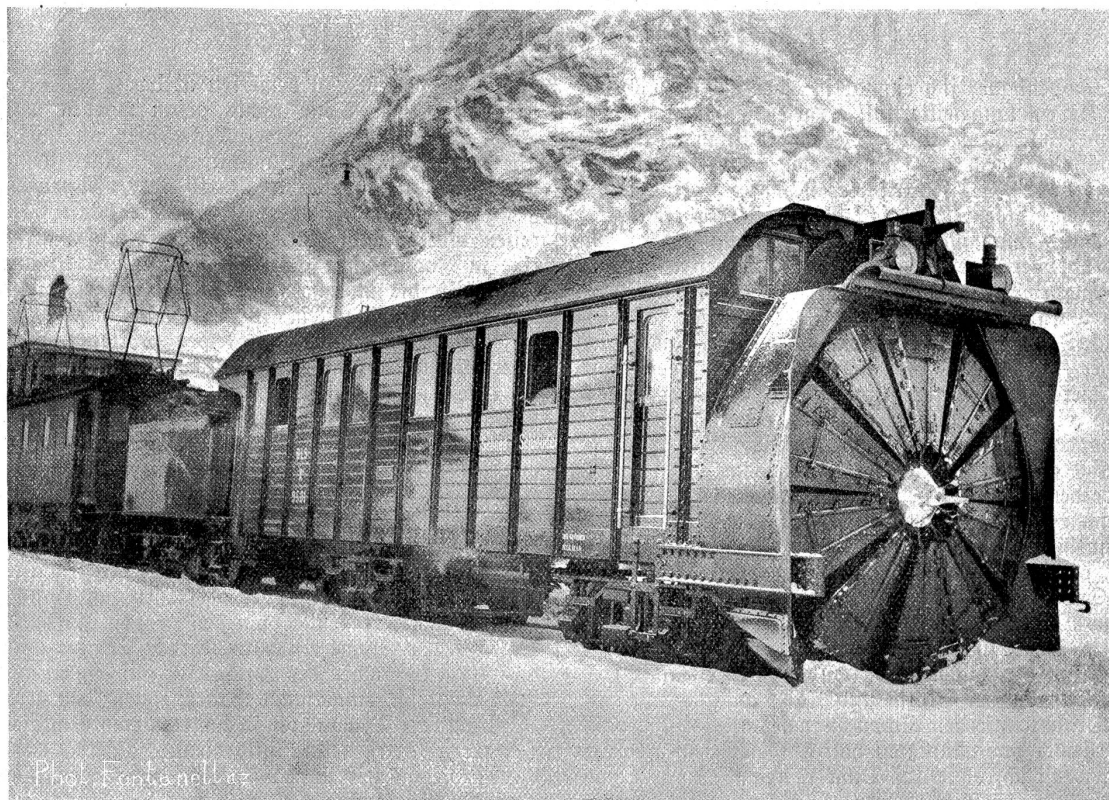
Die Schneeschleudermaschine der Lötchbergbahn.
