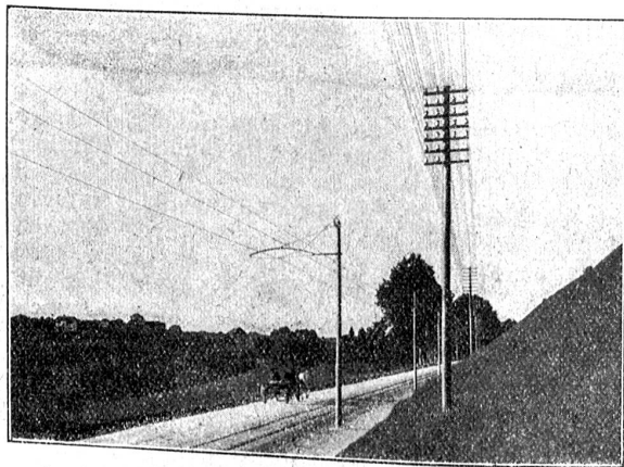
Abbildung 4. Sahnradtraher und Telephonleitung sind beide richtigerweise am aufsteigenden Rand der Straße aufgestellt; dagegen hätte das Crottoir an den Außenrand gehört. Durch die schwache Biegung des Auslegers gewinnt der Sahnradtraher an Gefälligkeit.
