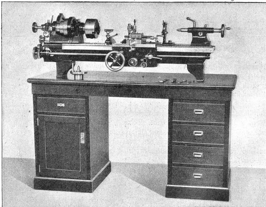
Leitspindel-drehbank
