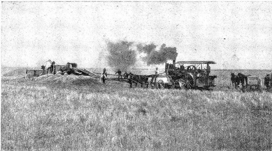
Dampfmaschine im Weizenfelde in Kansas. Der Drescher selbst wird mittelst eines langen, breiten Riemens von der Dampfmaschine getrieben.
