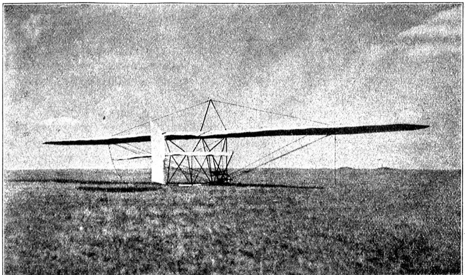
Flugzeug ohne Motor. Barth-Meijerschmitt-Eindecker mit verstellbarem Anstellwinkel der Tragflächen. Heute das erfolgreichste Segelflugzeug der Welt.
